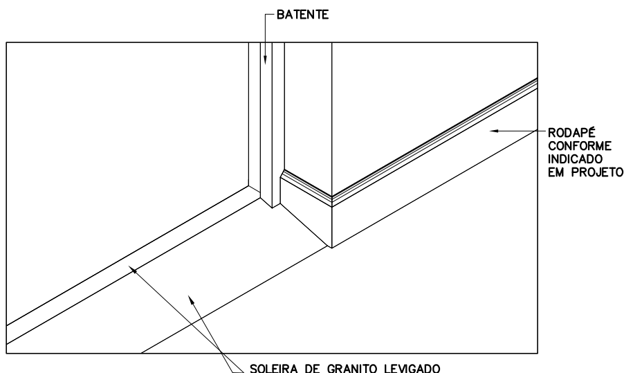
PERSPECTIVA ISOMÉTRICA SEM ESCALA
