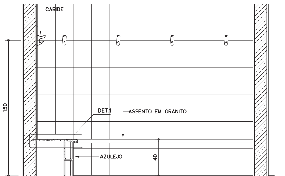
VISTA 1 ESC. 1:25
