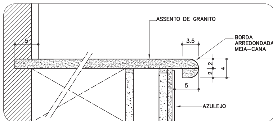
DETALHE 1 ESC. 1:5
