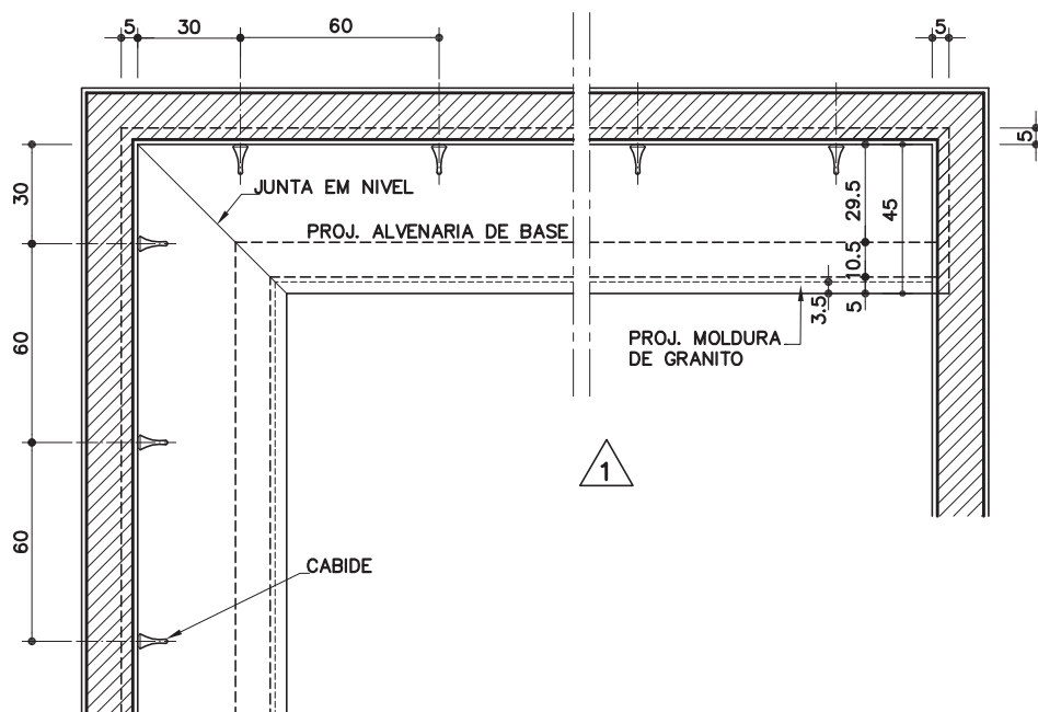
PLANTA ESC. 1:25
