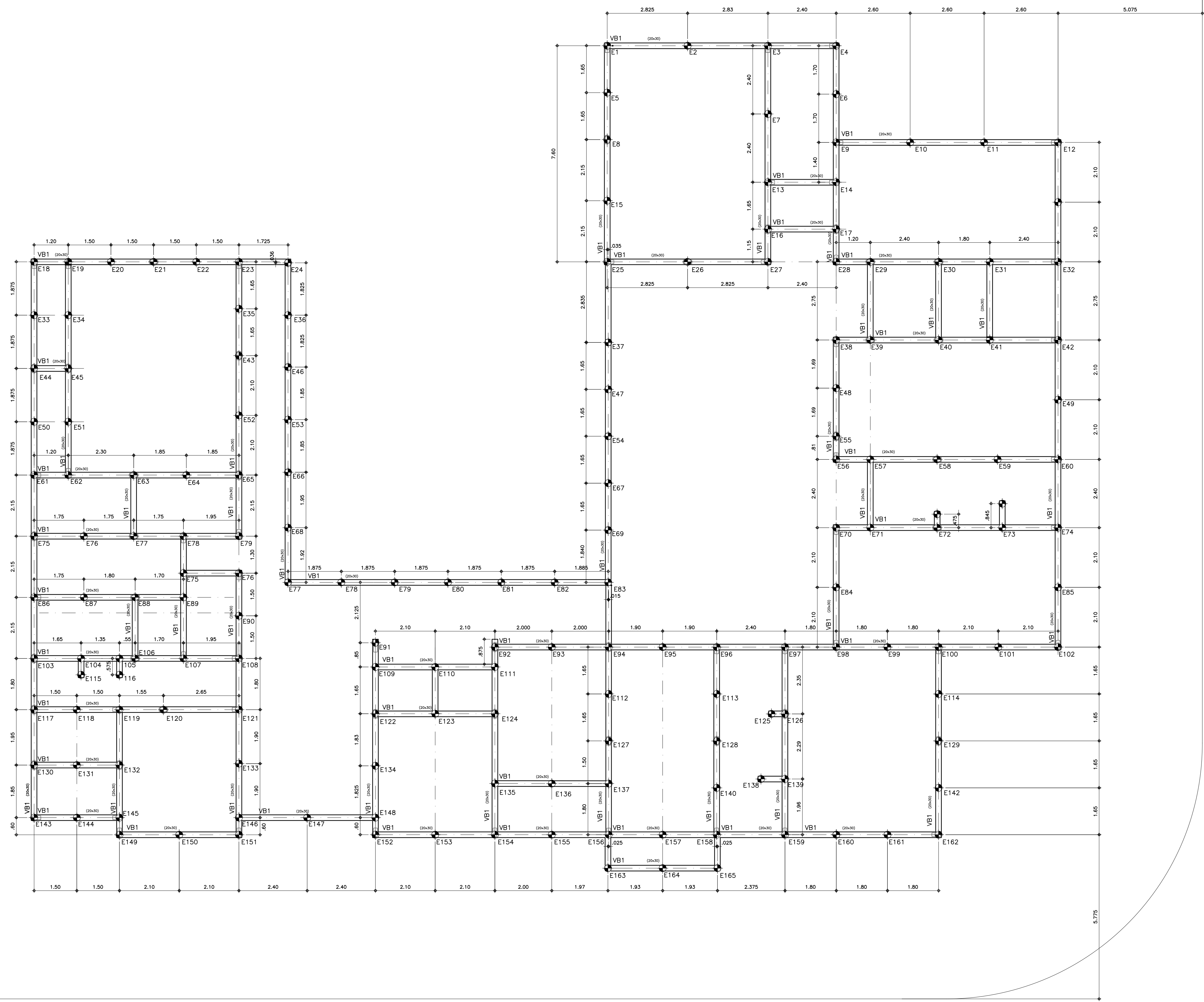
VIGAS BALDRAME ESC. 1:75
